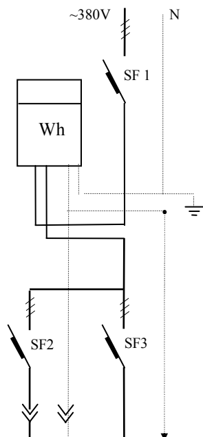
Elektros schema
