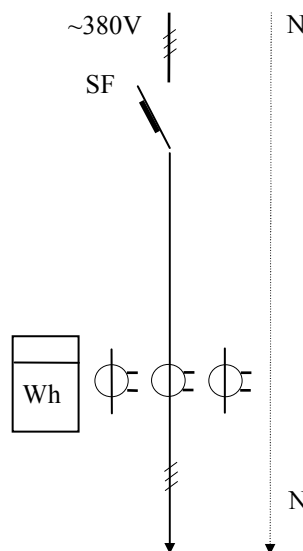
Elektros schema
